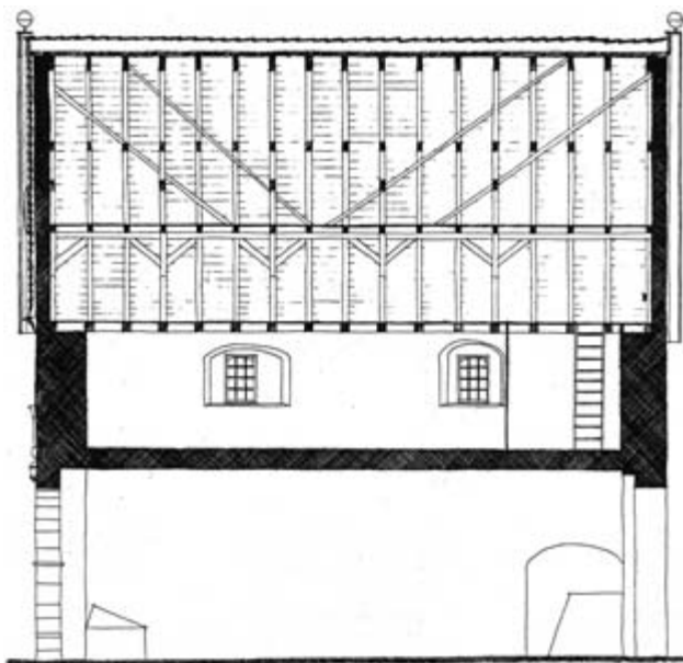
5. Snitt gjennom Stadspporten, tegnet av arkitekt Halfdan Wiberg i 1952. Det viser vaktstuen og loftet over hvelvingen.
