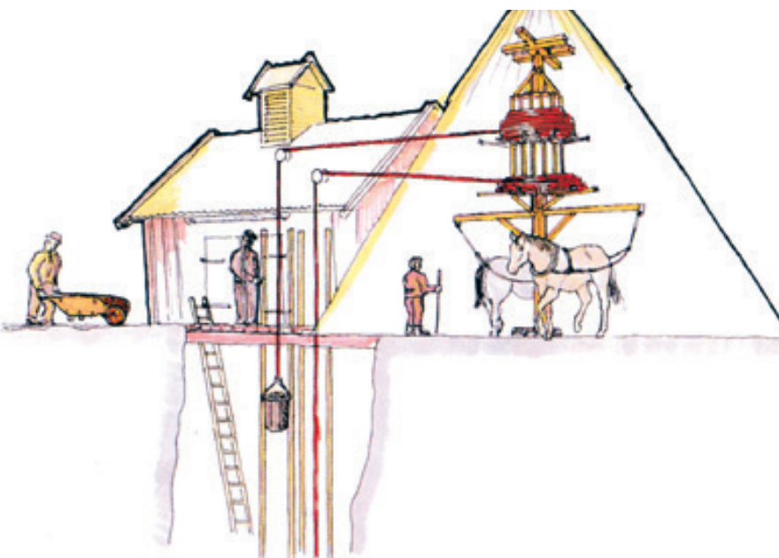
Heiseinnretning, såkalt hestegjøpel, til bruk i gruveanlegg. Tegning: Per J. Sagvolden.
